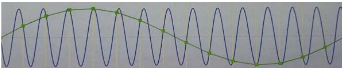
Slika 23. Poduzorkovanje ("Aliasing") [4]
