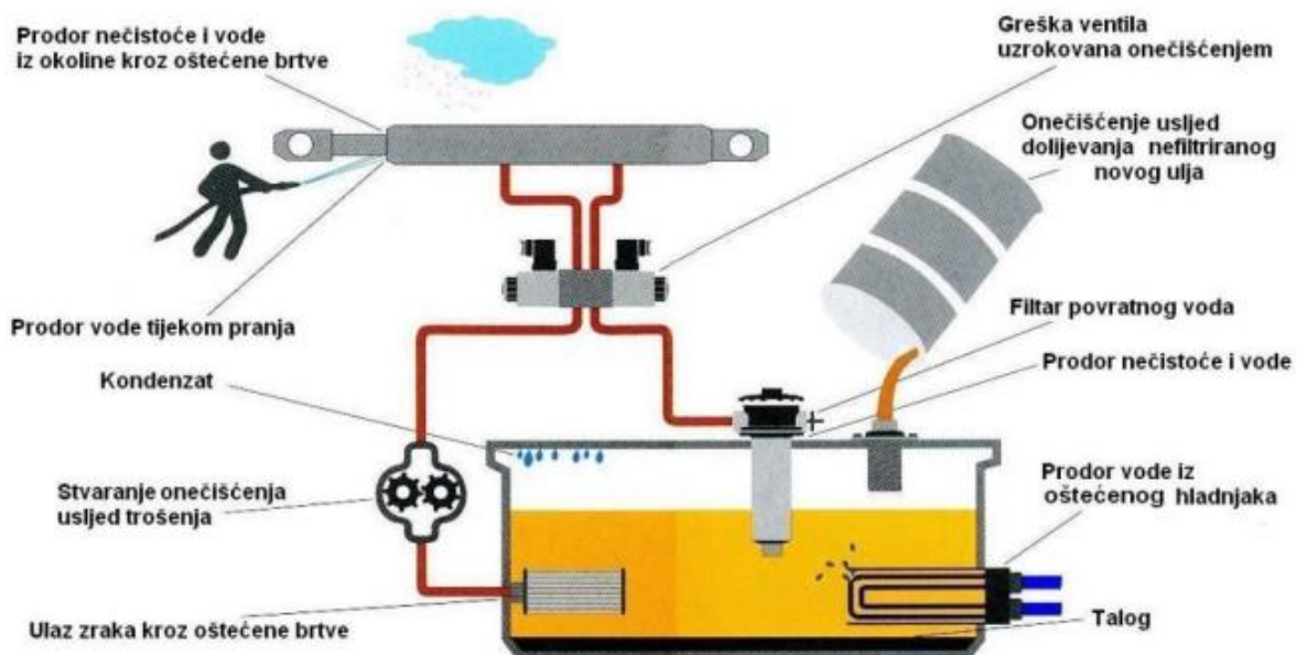
Slika 43. Onečišćenje ulja [36]
