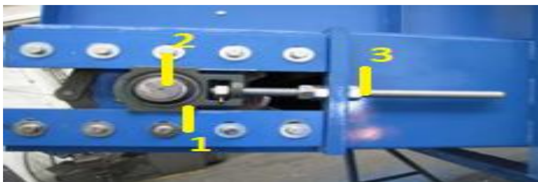
Slika 35. Zatezač lanca [13]
