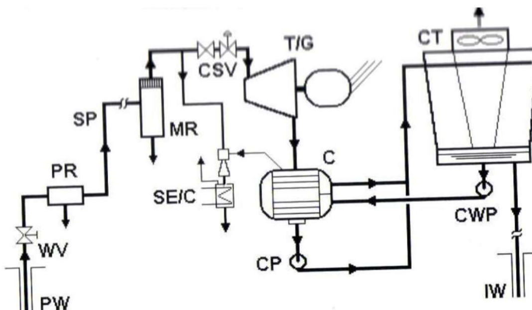
slika 2. Postrojenje sa suhom parom [8]
