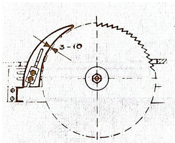
Slika 11: Razdvojni klin [9]
