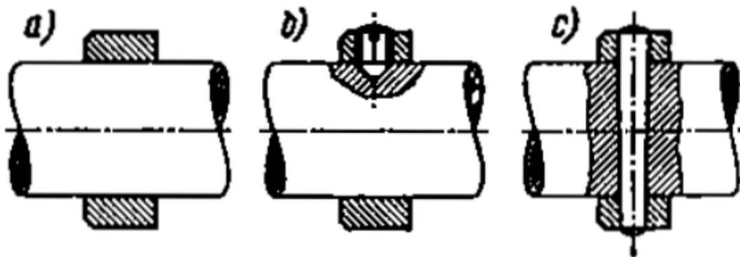
Slika 14. Prstenovi kao ojačanja vratila [2]
