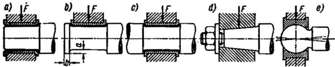
Slika 13. Nosivi rukavci [2]
