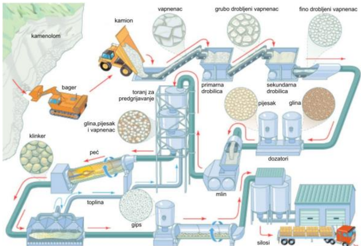
Sl. 3 Suvremeni način proizvodnje cementa [2]
