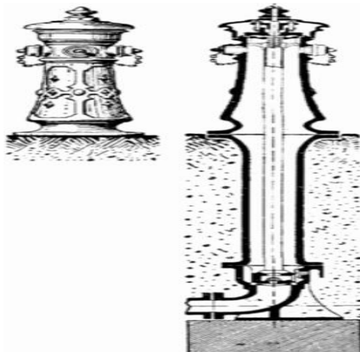
Slika 6. Stariji model nadzemnog hidranta[10]
