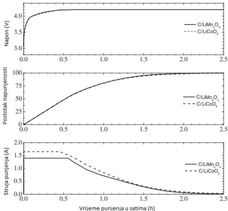
Slika 13. Napon, stanje napunjenosti i struja punjenja 18650 ćelije. Izvor [14].
