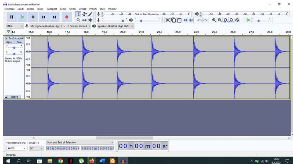
Slika 17. Predodžba snimljenog audio zapisa bas bubnja u Audacity programu
