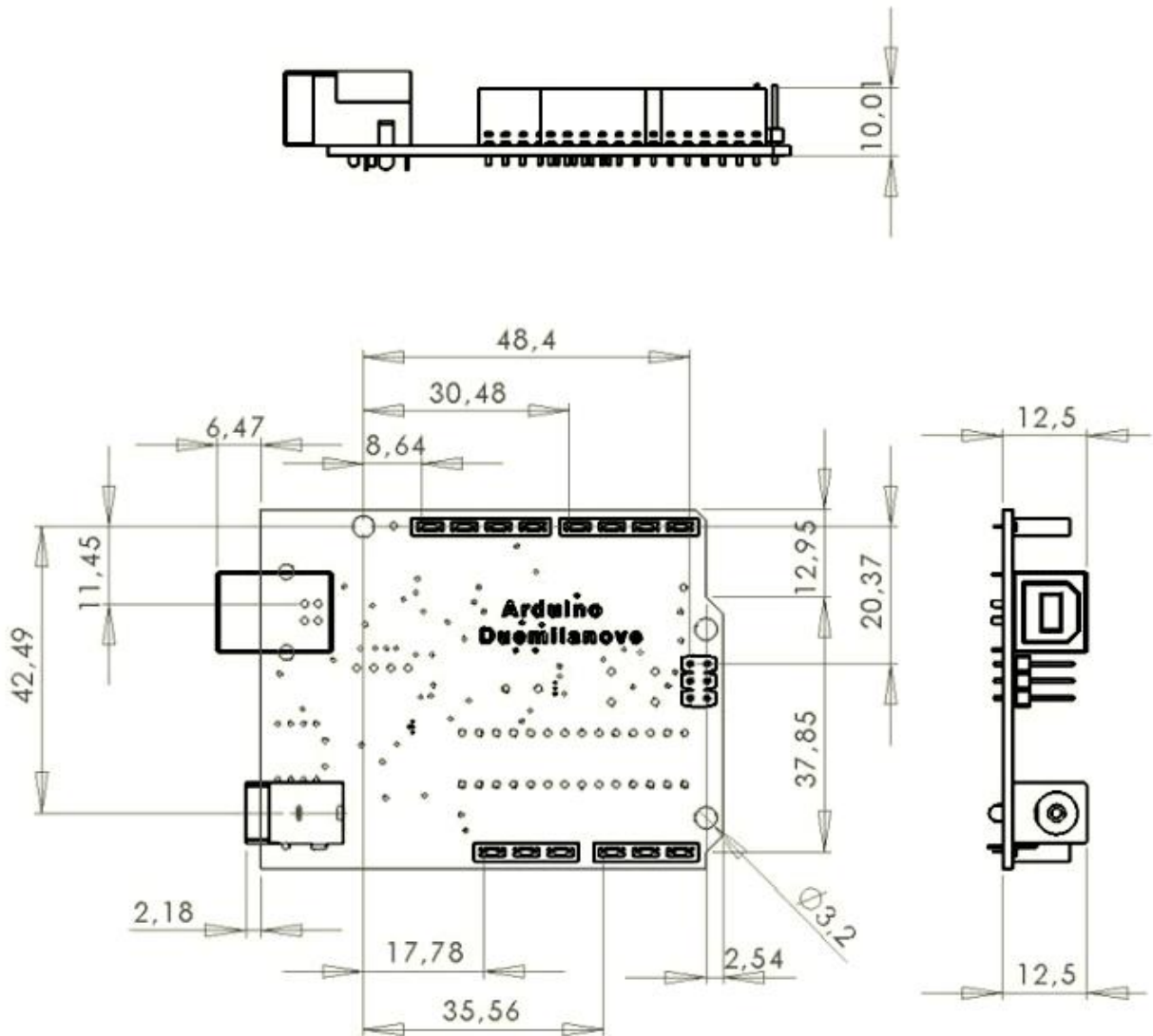
Slika 3. Predodžba dimenzija mikro upravljača Arduino UNO [12].
