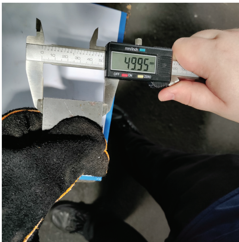
Slika 26.: Mjerenje druge dimenzije pomičnim mjerilom
