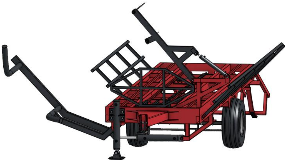
Slika 36. Princip istovara tereta preko stražnje rampe
