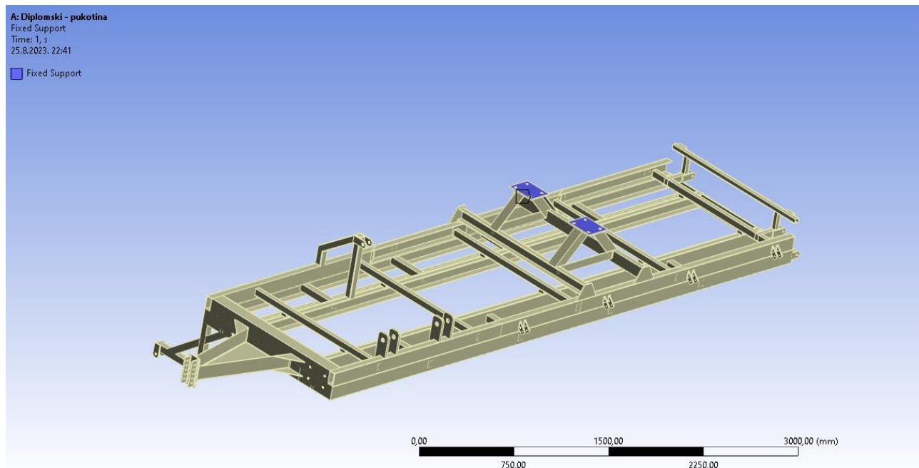
Slika 22. Plave površine označavaju "fixed support" odnosno povezanost prikolice s okolinom preko osovine i nosača osovine
