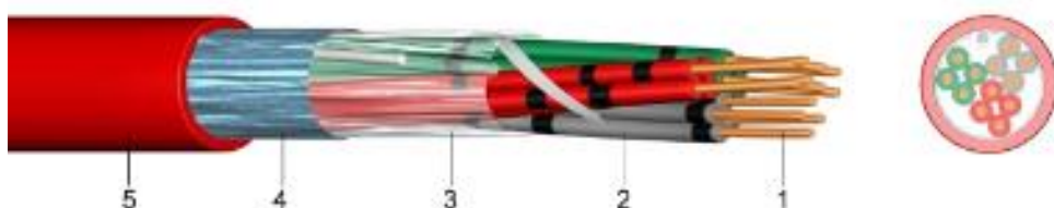
Slika 40. Vatrodojavni kabel [21]
