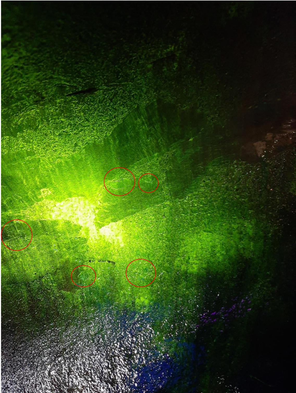
Indikacije na reparaturnom zavaru ispod kućišta brtvi
