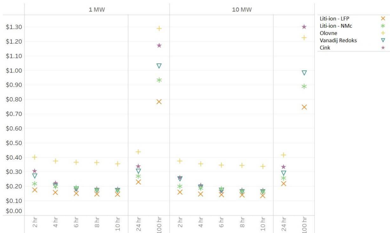
Slika 26 LCOS troškovi ($/kWh) u 2030. godini za 1-10MW sustave [5]
