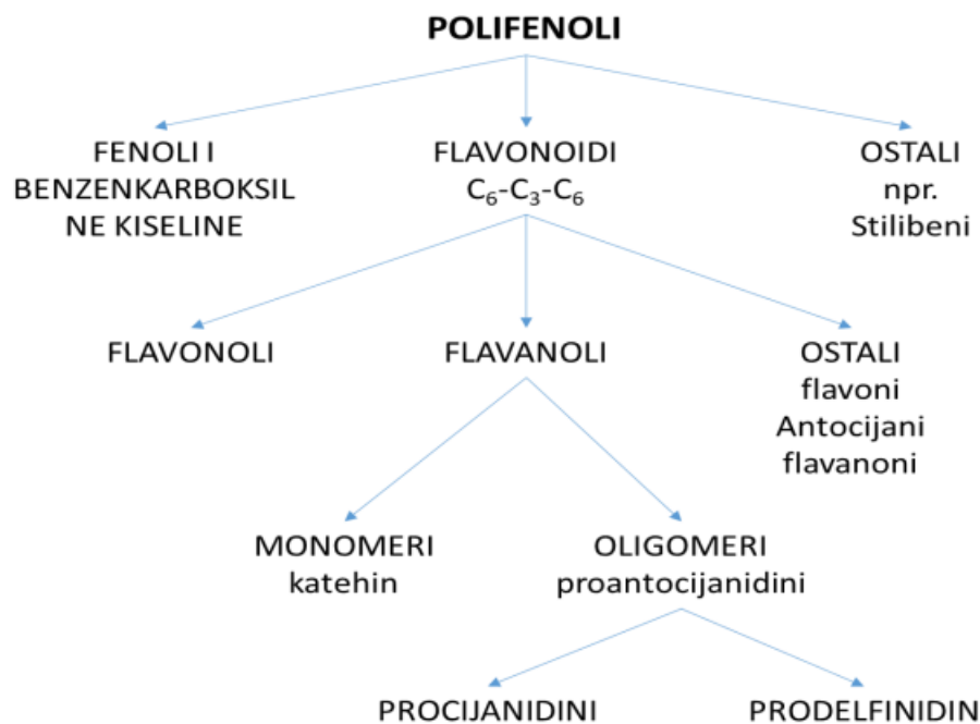
Slika 13. Osnovna podjela polifenola (Berend i Grabarić, 2008).
