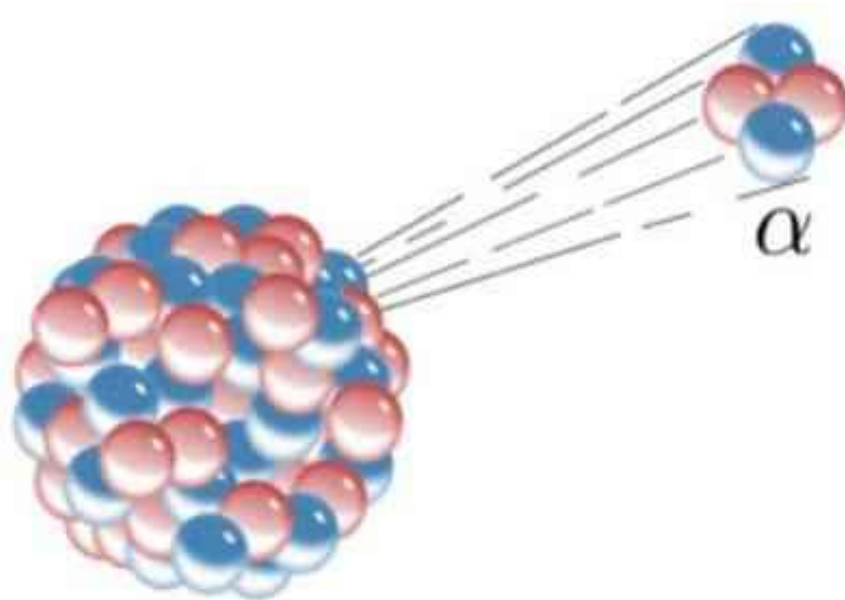
Slika 2: Slikoviti prikaz alfa zračenja [3]
