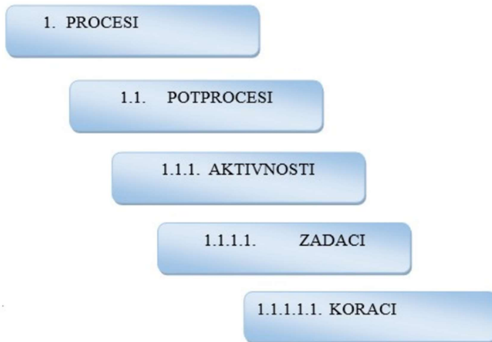
Slika 4. Hijerarhija procesa
