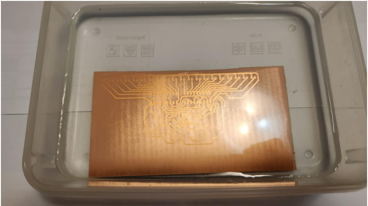
Slika 54. Tiskana pločica u tijeku postupka jetkanja
