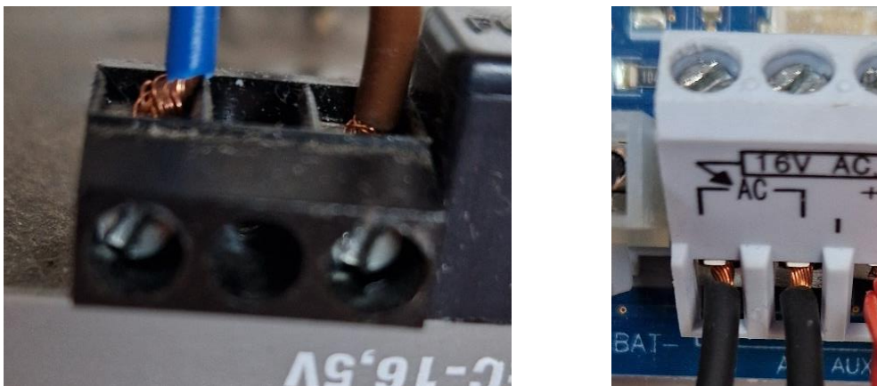
Slika 30. Spajanje transformatora
