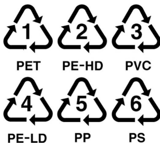
Slika 1. Plastomeri [2].
