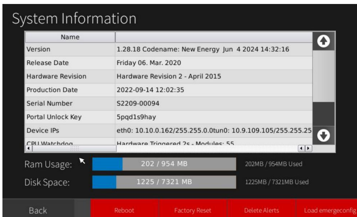
Slika 27. Prikaz modula „Information“ [Autor: Karlo Ivešić]
