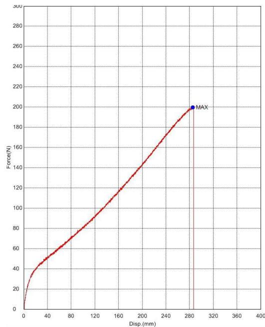
Slika 36. Dijagram sile / produljenje za epruvetu 2
