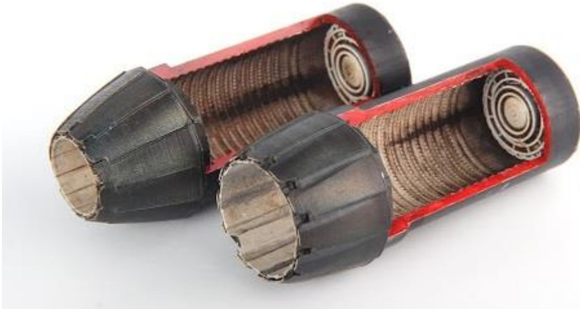
Slika 8. Ispušna mlaznica F404 [8]
