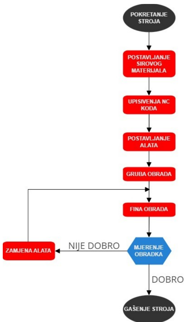
Slika 5. Dijagram toka kod procesa glodanja [6]
