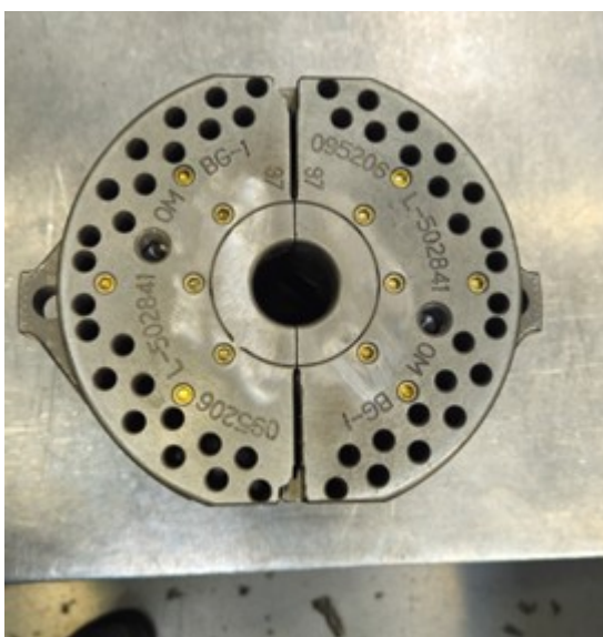
Slika 59. Izgled kalupa
