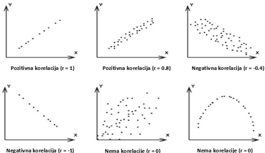
Slika 6. Dijagram raspršenja [6]
