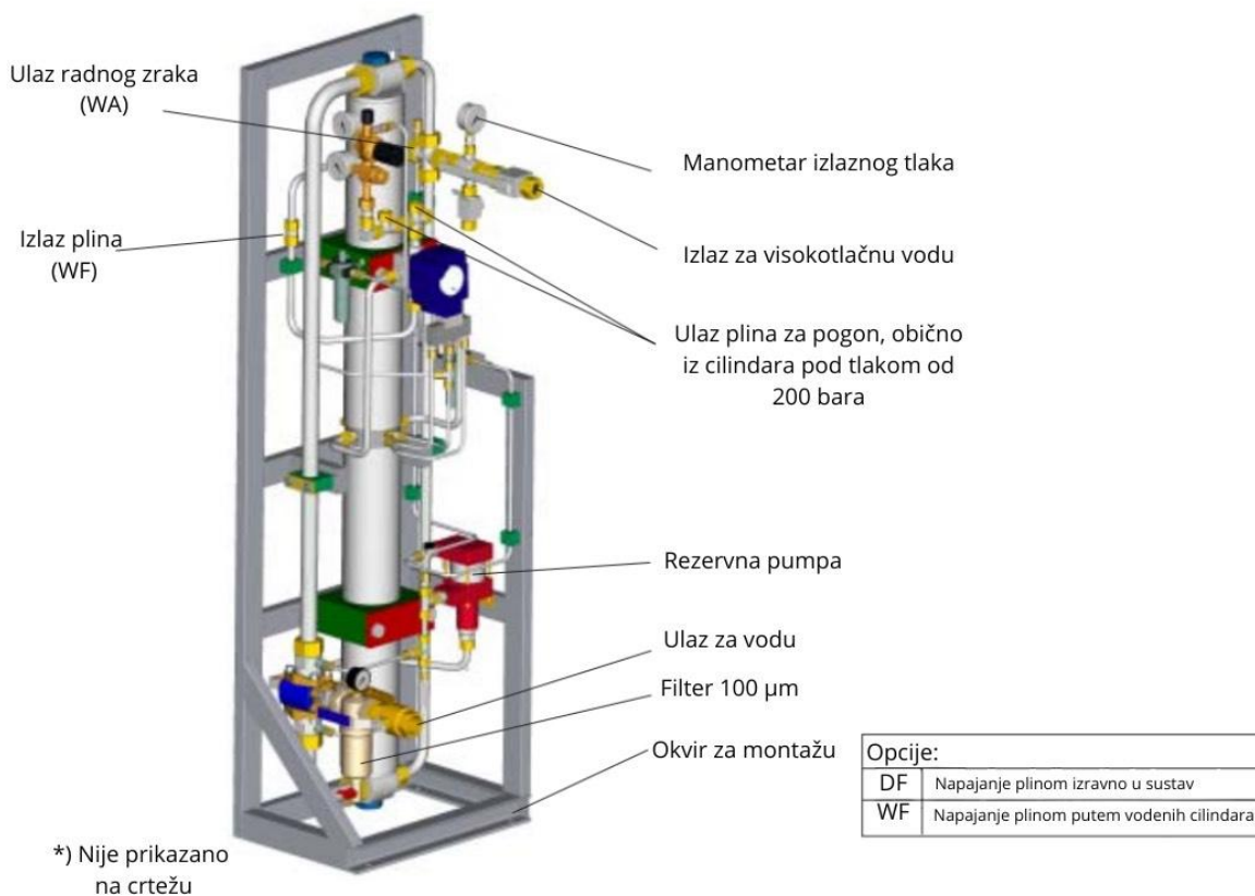
Slika 13. GPU [10]
