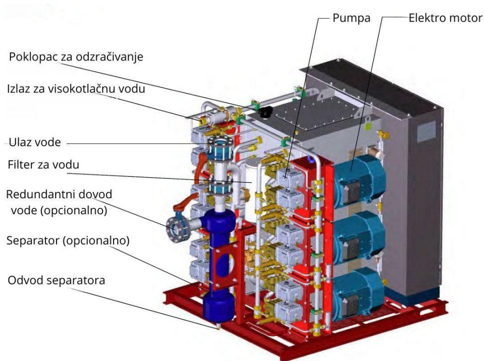
Slika 11. BPU [8]
