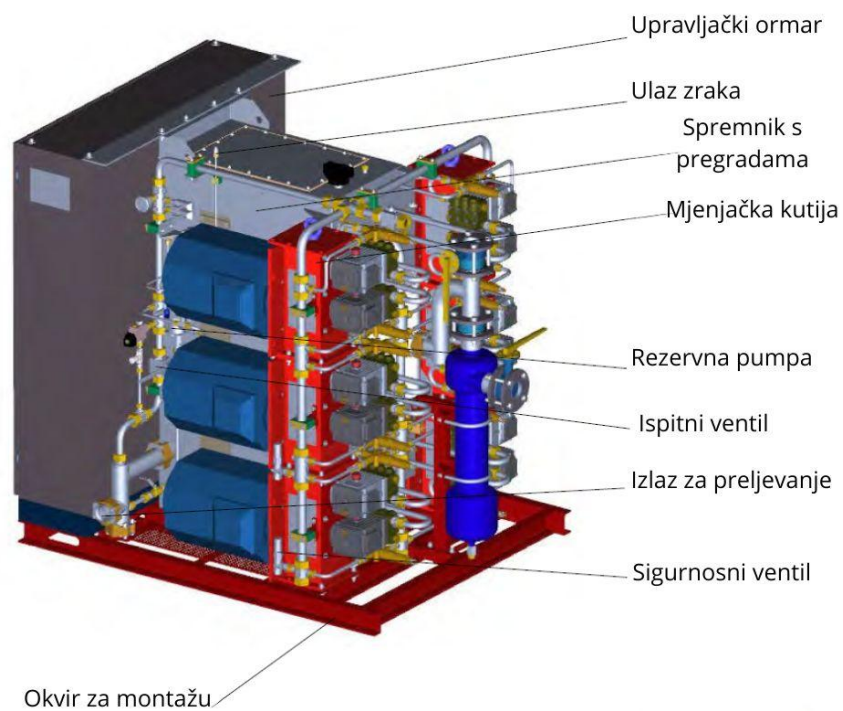
Slika 8. SPU [8]
