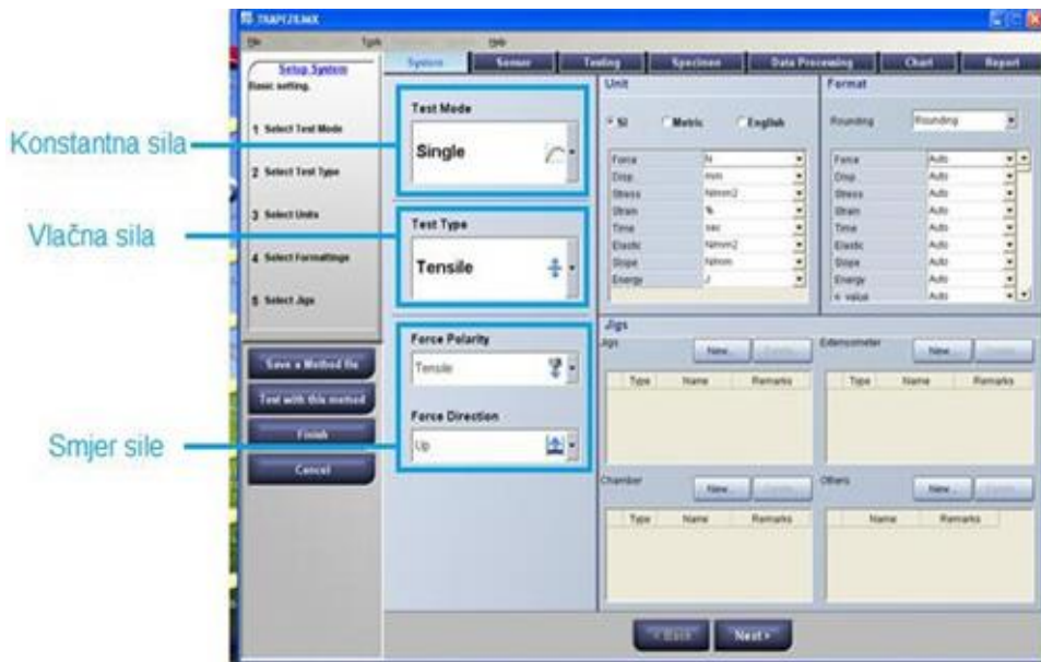
Slika 53. Odabir sile
