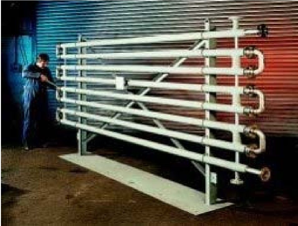
Slika 38. Izmjenjivač topline s dvostrukom cijevi
