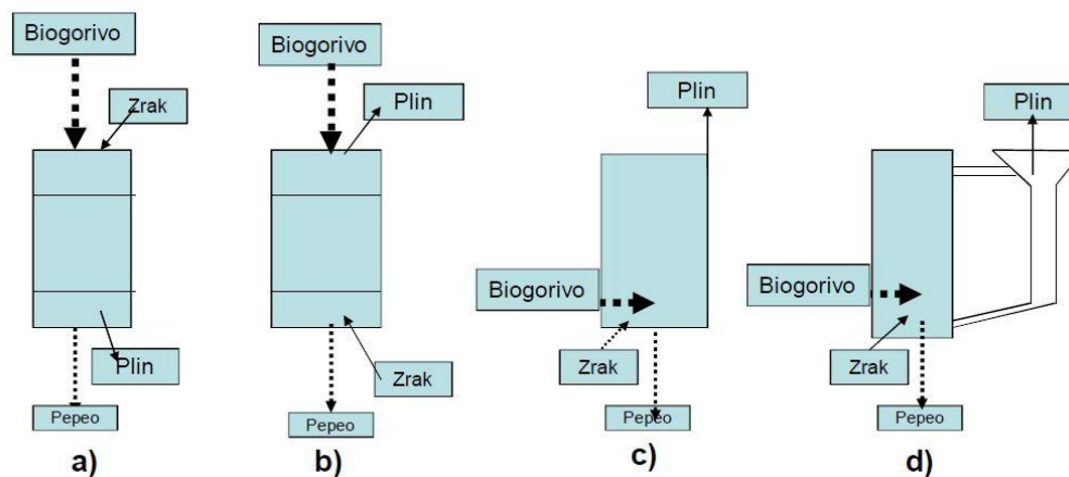
Slika 10 . Podjela rasplinjača
