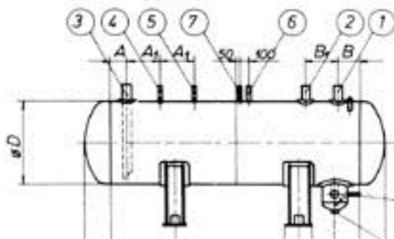
Slika 13. Sakupljač tekućine (rezervoar)
