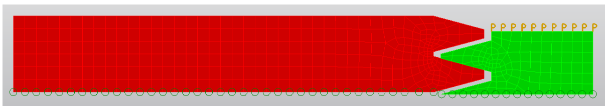
Slika 38 - Rubni uvjeti na vretenu
