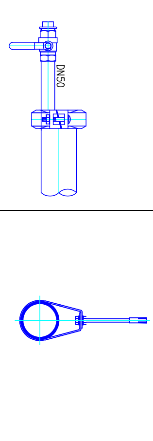
Detalj 1: Priključak za sprinkler
