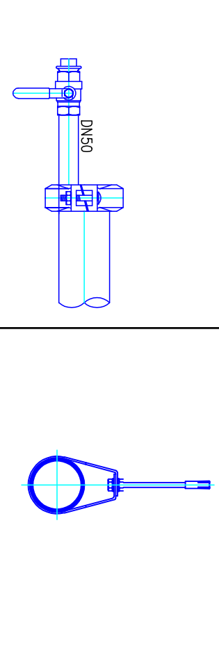
Detalj 1 Priključak za sprinkler
