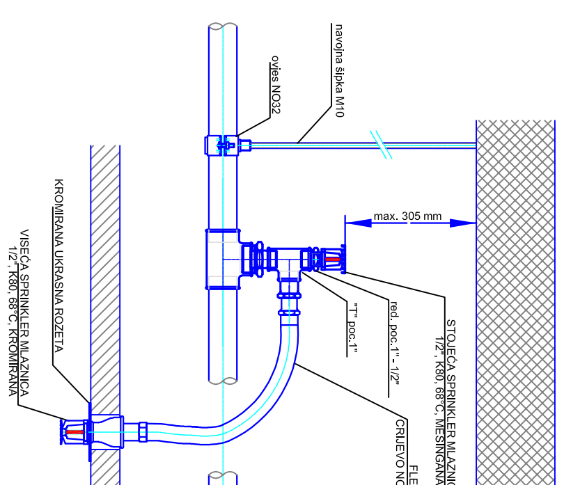
Detalj 4 DETALJ UGRADNINE SPINKLERI VEŠICE MALIŠNE
