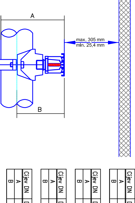
Detalj 2 Detalj priključka
