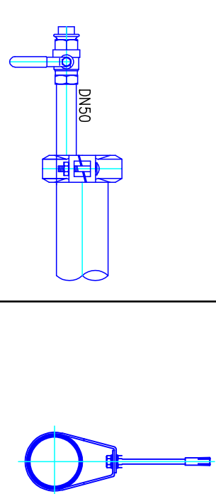
Detalj 1 Priključak za špičanje
