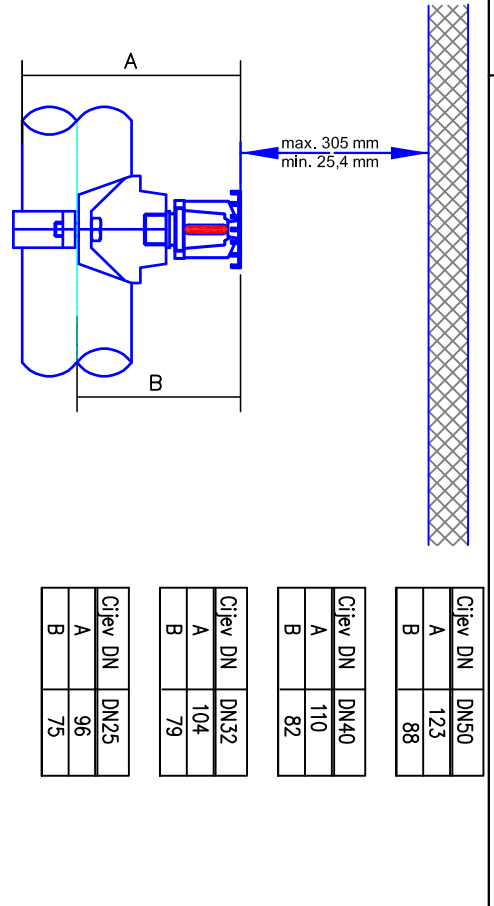
Detalj 2 Detalj uređaja sprinkler visoke mlaznice
