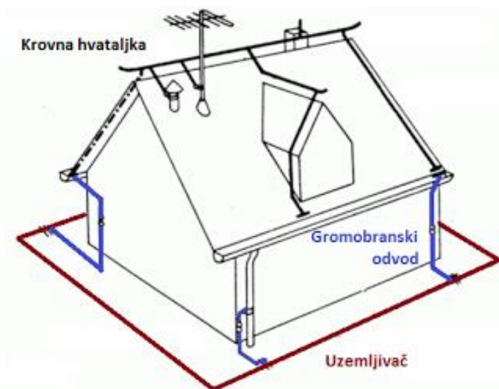
Slika 11. Gromobranska instalacija
