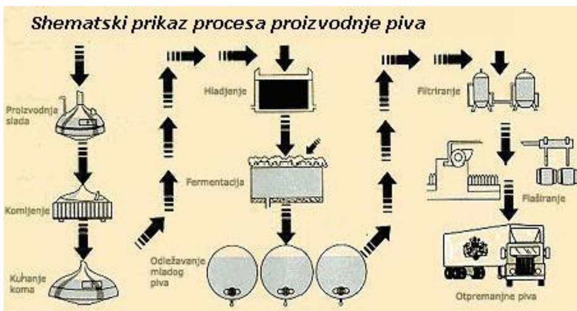
Slika 1. Shema proizvodnje piva. Izvor: http://www.pinta.hr/o_pivu/izrada_piva.html
