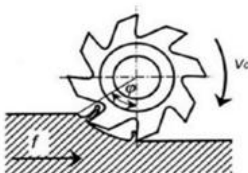
Slika 3. Obodno glodanje
