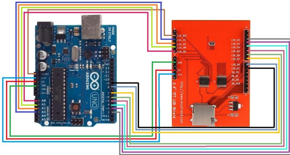
Slika 11. Predodžba povezivanja LCD ekrana na Arduino ploču
