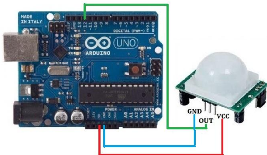
Slika 13. Predložba spajanje osjetila pokreta sa Arduino pločom
