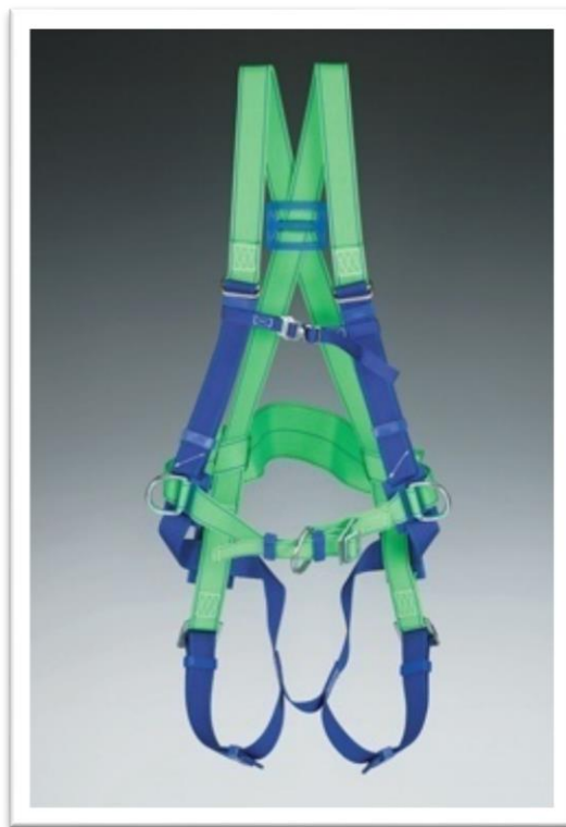
Slika 8. Zaštitni pojas za cijelo tijelo s karakterističnim spojnim "D" prstenima
