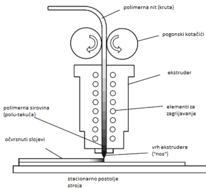
Slika 3. FDM postupak. [3]
