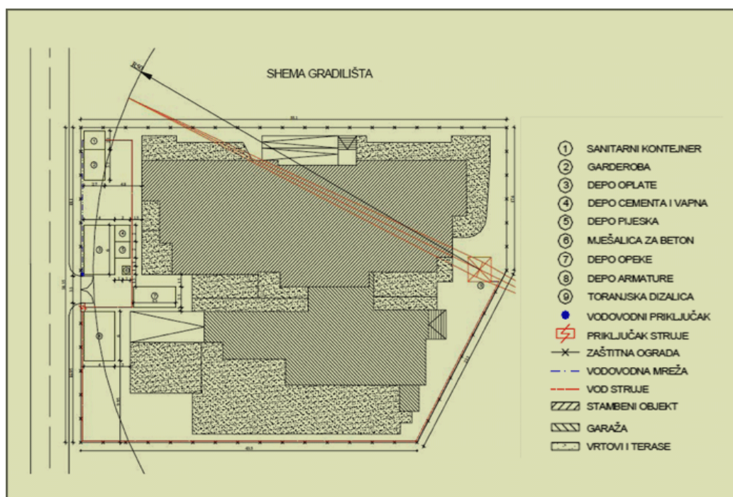
Slika 1. Shema gradilišta
