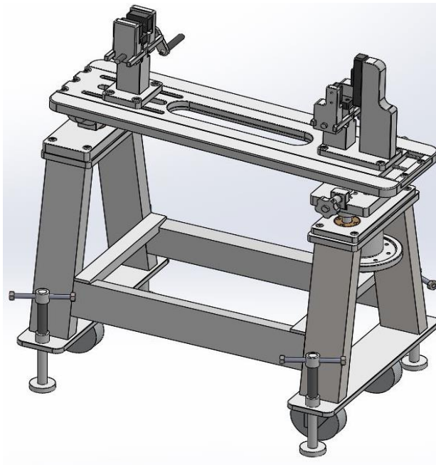
Slika 34. Gotova naprava
