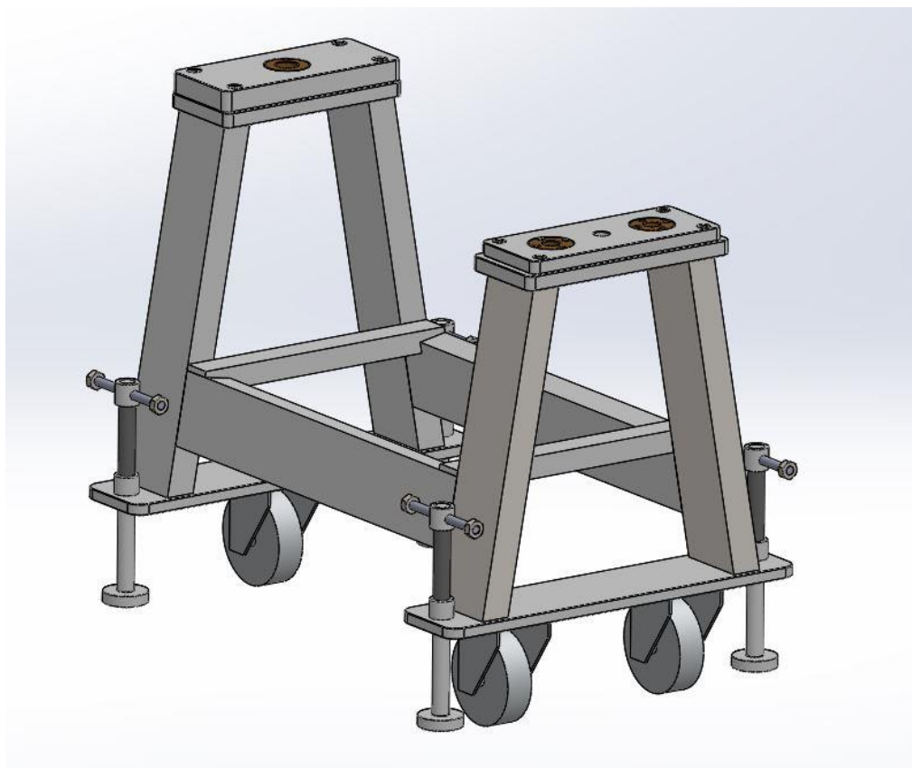
Slika 33. Postolje naprave
