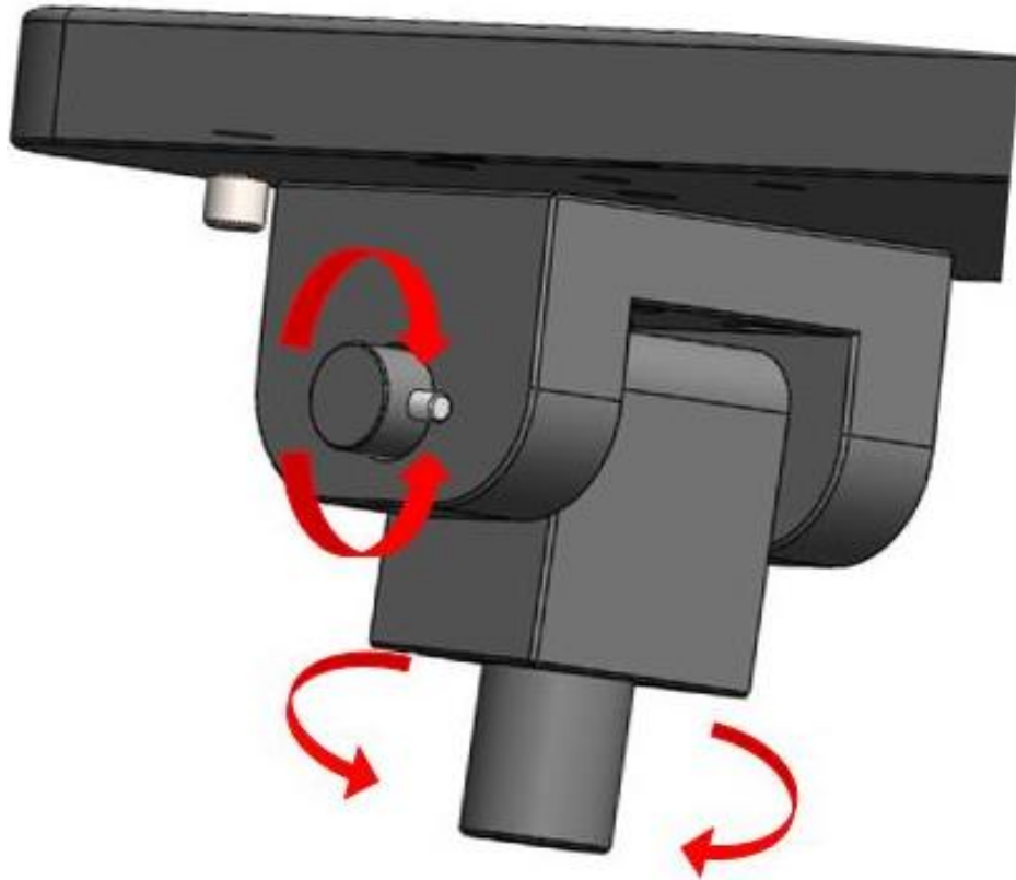
Slika 23. Prednji zglob
