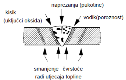
Slika 2. Prikaz najčešćih grešaka zavrenog spoja na Al materijalima
