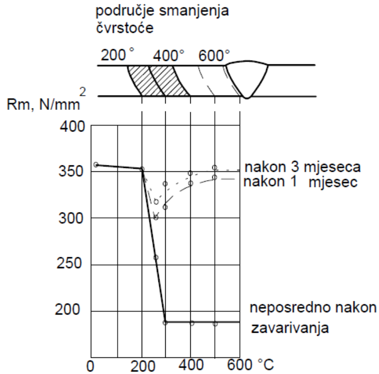
Dijagram 1. Ovisnost vlačne čvrstoće o promjeni temperature
