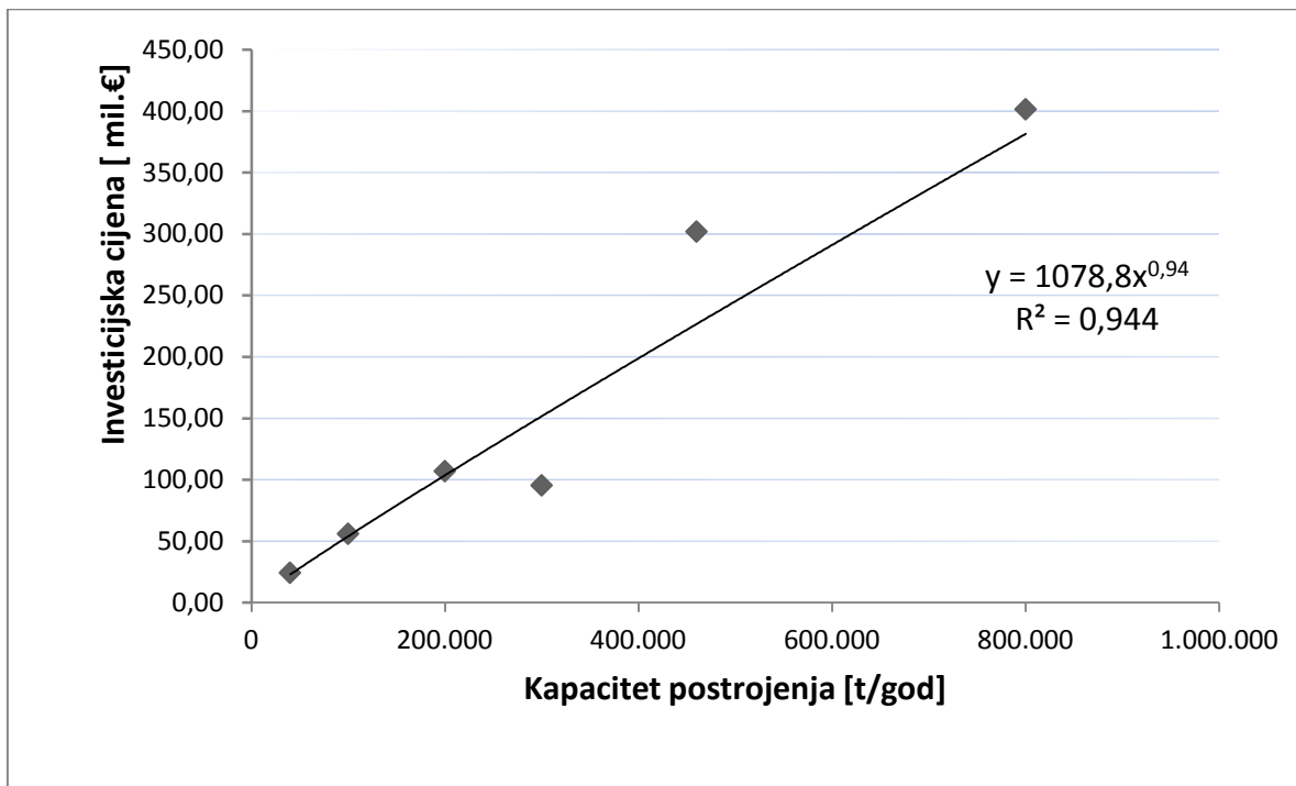
Slika 16. Ovisnost investicijskih troškova o veličini postrojenja
