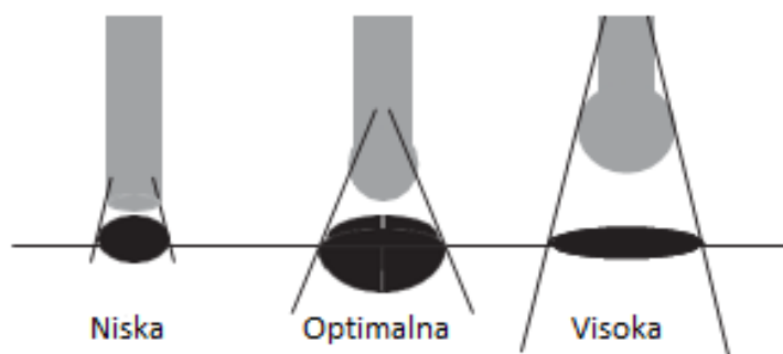
Slika 15. Podešavanje oblika izgleda zavora osnovnom strujom zavarivanja [11]
