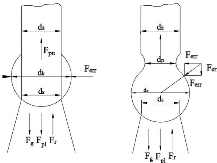
Slika 3. Djelovanje sila na kapljicu metala u električnom luku [4]
