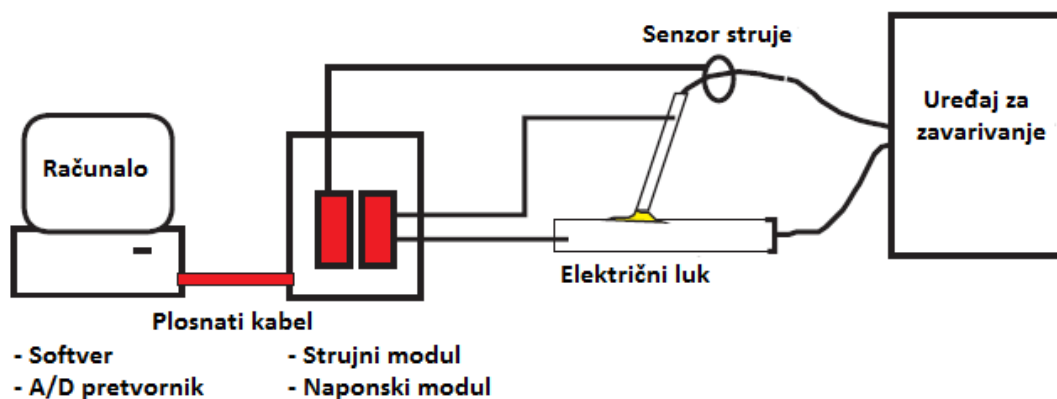
Slika 17. Shematski prikaz Online sustava za praćenje glavnih parametara zavarivanja [13]
