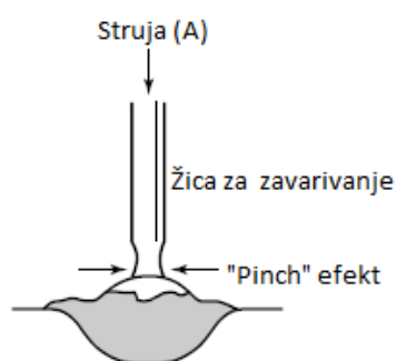
Slika 6. Shematski prikaz pojave "pinch" efekta [3]
