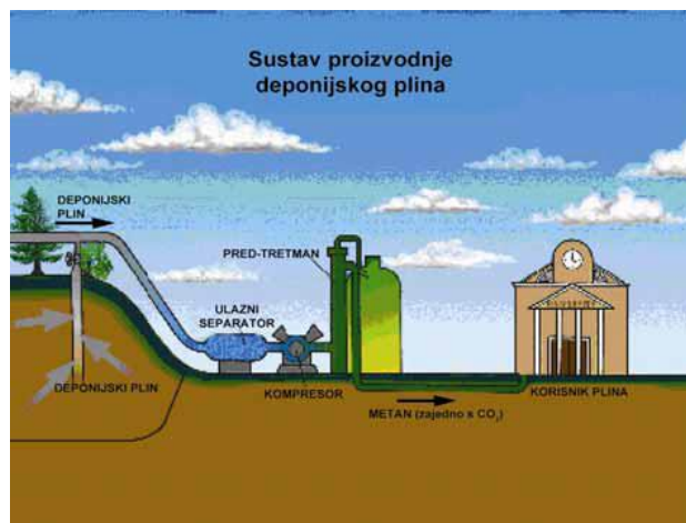
Slika 42: Sustav za prikupljanje i iskorištavanje deponijskog plina
