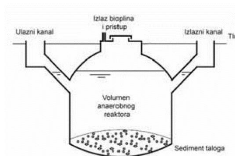
Slika 35: Kineski reaktor za fermentaciju
