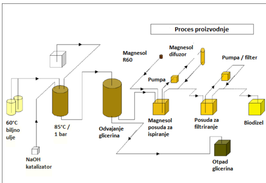
Slika 25: Pojednostavljeni prikaz ciklusa proizvodnje biodizela
