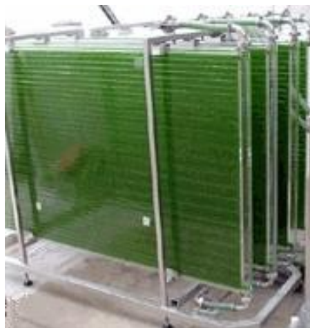
Slika 12: Zatvoreni sustav uzgoja algi
