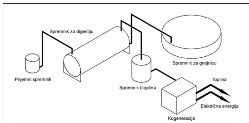
Slika 37: Shematski prikaz bioplinskog postrojenja na poljoprivrednim gospodarstvima
