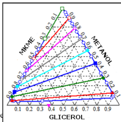
Slika 18: Dijagram mješavine MKME-metanol-glicerola pri tlaku od 1 bar
