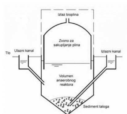
Slika 36: Kineski reaktor za fermentaciju
