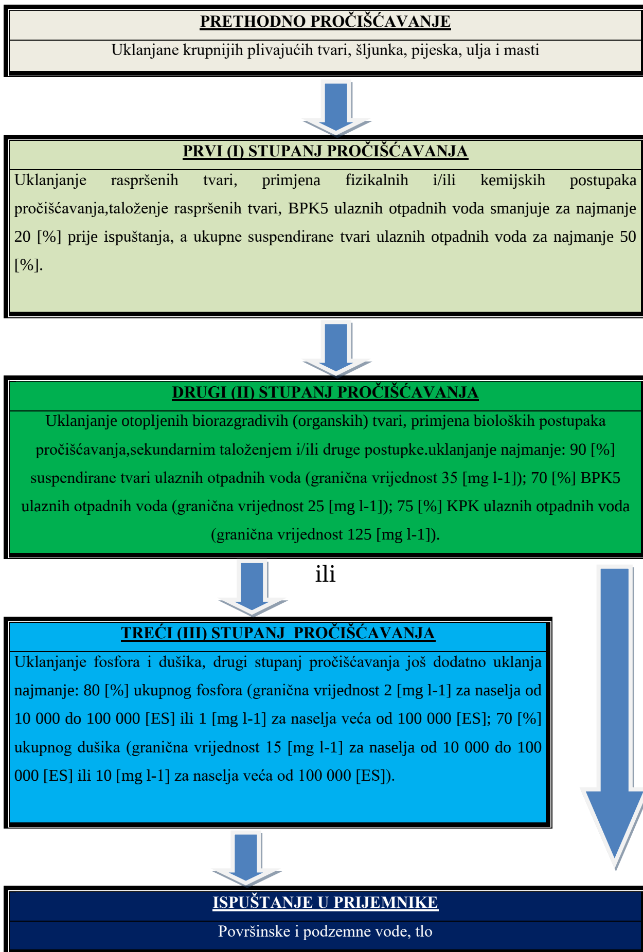
Slika 5 Procesi pročišćavanja otpadnih voda
