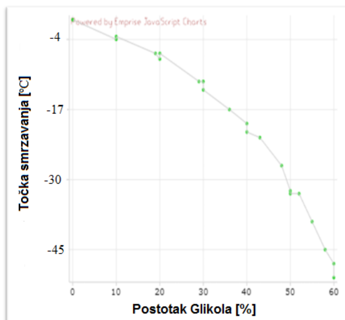
Slika 39. Točka smrzavanja u ovisnosti o postotku glikola u radnoj tvari.
