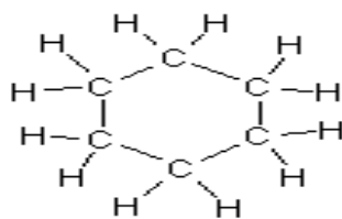
Slika 11. Cikloheksan
